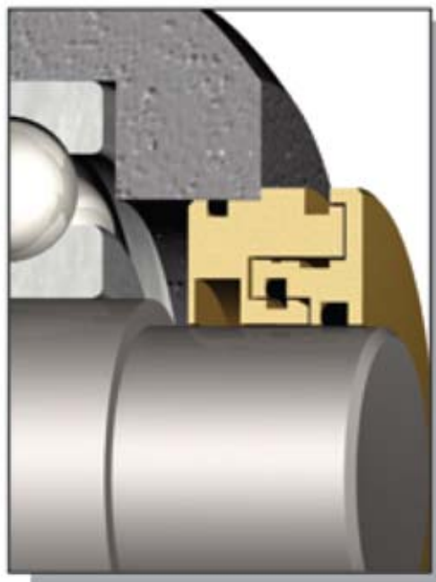
Inpro/Seal® VBXX-D
